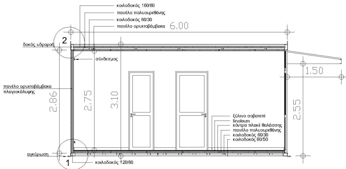
ΤΟΜΗ Β-Β
