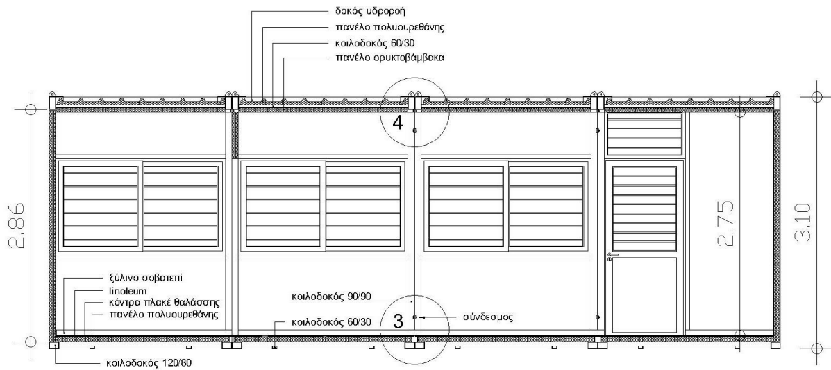
ΤΟΜΗ Α-Α
