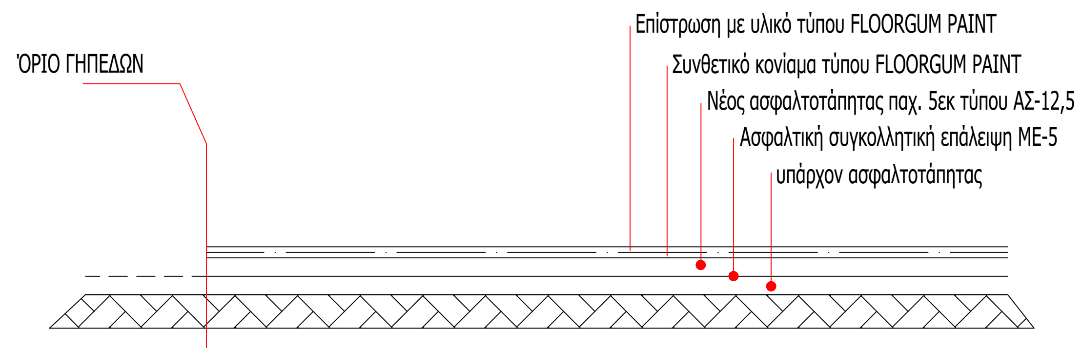
ΤΟΜΗ ΣΤΗΝ ΘΕΣΗ ΤΩΝ ΓΗΠΕΔΩΝ κλίμακα 1:10
