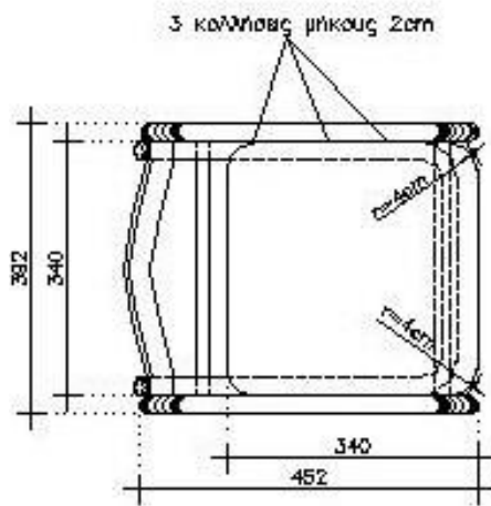
ΚΑΤΩΨΗ ΚΑ. 1:10
