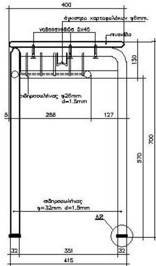
ΠΛΑΓΙΑ ΟΨΗ ΚΑΤΑΣΚΕΥΗ 1:6
