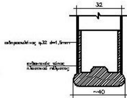
ΛΕΙΠΤΟΜΕΡΕΙΑ Δ1
