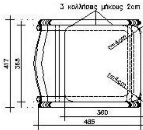
ΚΑΤΟΨΗ ΚΛ. 1:10
