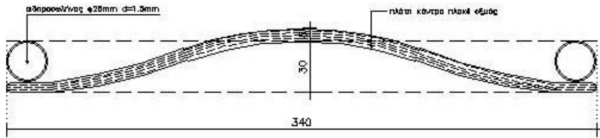
ΤΟΜΗ ΚΟΝΤΡΑ ΠΛΑΚΕ ΠΛΑΤΗΣ ΚΑΙΜΑΚΑ 1:20
