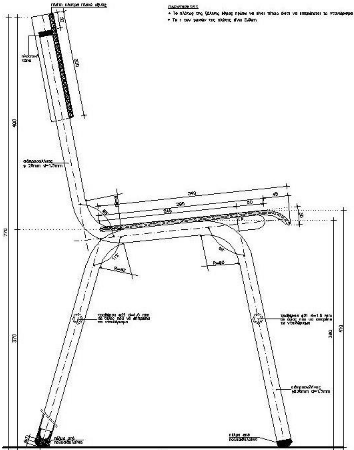
ΚΑΘΙΣΜΑΤΑ ΤΡΑΠΕΖΟΘΡΑΝΙΩΝ ΜΕΤΑΛΛΙΚΑ ΔΗΜΟΤΙΚΟΥ Νο4
