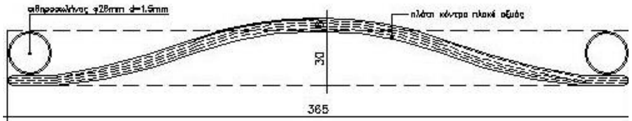
ΤΟΜΗ ΚΟΝΤΡΑ ΠΛΑΚΕ ΠΛΑΤΗΣ ΚΛΙΜΑΚΑ 1:20
