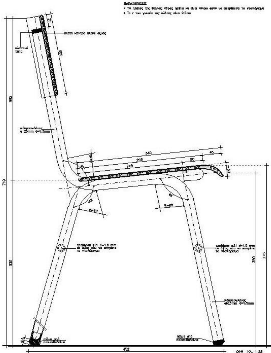
ΚΑΘΙΣΜΑΤΑ ΤΡΑΠΕΖΟΘΡΑΝΙΩΝ ΜΕΤΑΛΛΙΚΑ ΔΗΜΟΤΙΚΟΥ Νο3
