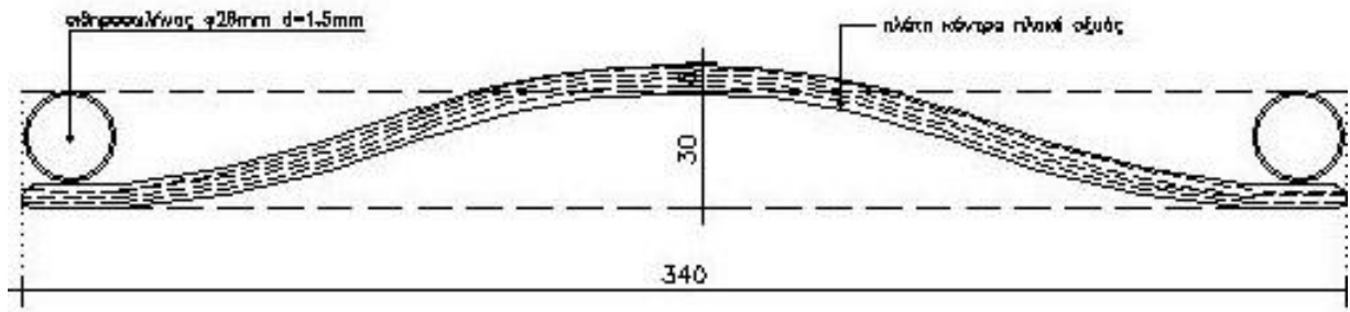
ΤΟΜΗ ΚΟΝΤΡΑ ΠΛΑΚΕ ΠΛΑΤΗΣ ΚΛΙΜΑΚΑ 1:20
