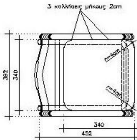
ΚΑΤΩΨΗ ΚΛ 1:10
